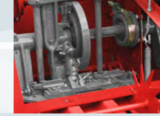
TELLİ BAĞLAMA GRUBU
