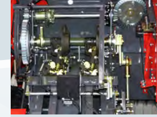
2 İPLİ BAĞLAMA GRUBU
