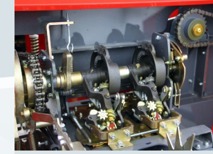
RASSPE BAĞLAMA TİPİ
